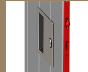
SERRURE CENTRALE À ROULEAU
