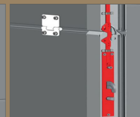
SERRURE À CROCHETS HAUTE ET BASSE
